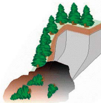
「深層崩壊」
