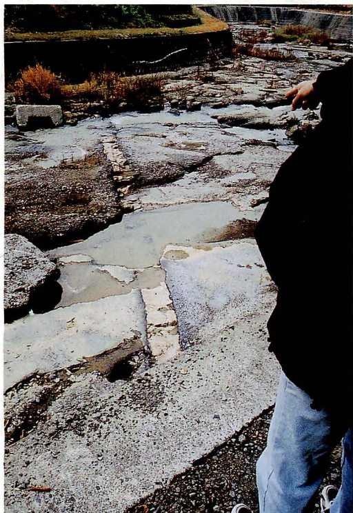
▶ 清水橋の上流の表川にある礫岩の中に入った変成岩
