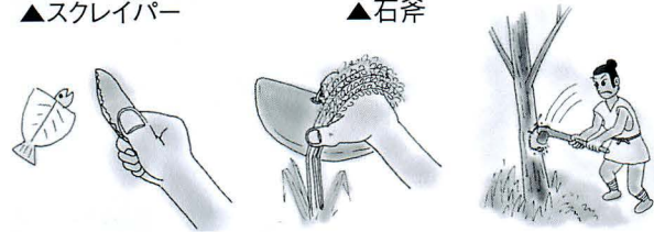
▲スクレイパー
