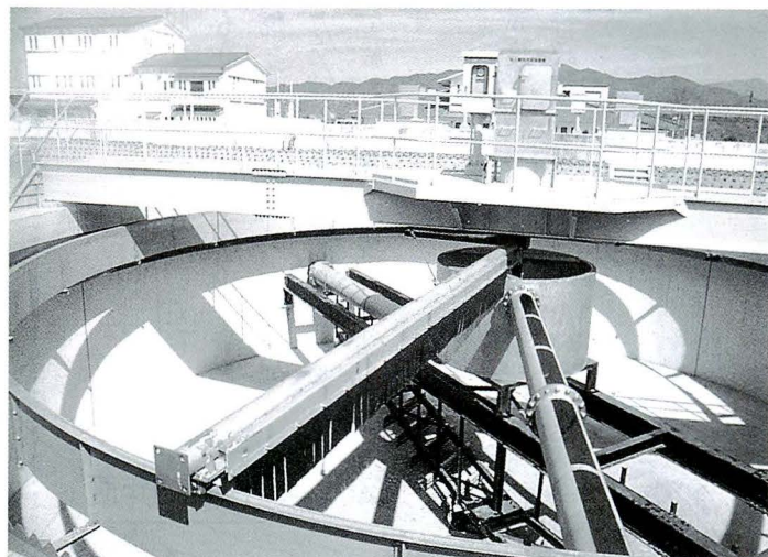
①最終沈殿池
